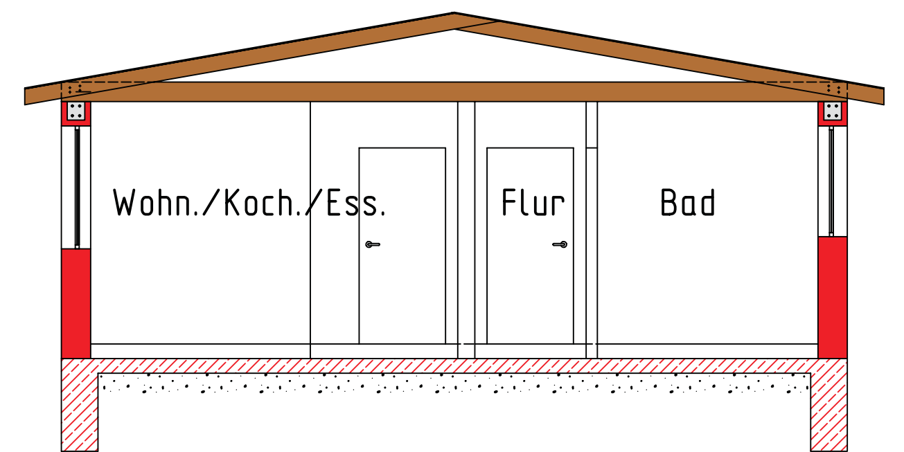
Schnitt A-A
